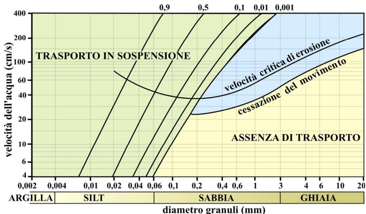
Fig. 8 - Relazione tra velocità dell'acqua e granulometria. La curva della velocità critica di erosione indica la velocità minima affinché inizi il prelievo di materiale. La movimentazione è più facile con grani intorno a 0,2 mm rispetto a quelli più piccoli, fra loro più coesi. Con il materiale è in movimento è sufficiente una velocità inferiore affinché avvenga la cessazione del movimento . I valori sulla parte superiore del diagramma si riferiscono alle curve della concentrazione relativa del trasporto solido , rapporto tra la torbidità a metà altezza tra superficie e fondo e quella in corrispondenza del fondo.
